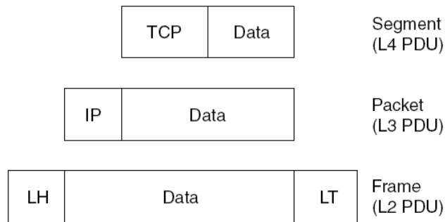
Gambar 2.18 Frame, Paket dan Segmen
