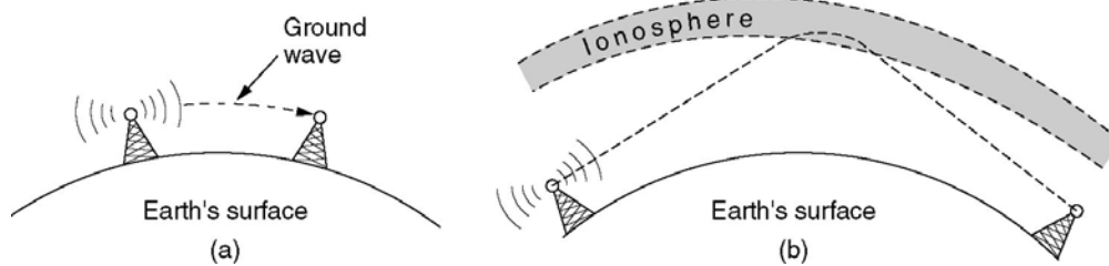
Gambar 3.31 Komunikasi radio
