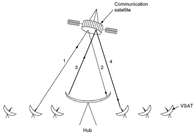
Gambar 3.35 Komunikasi satelit dengan VSAT
