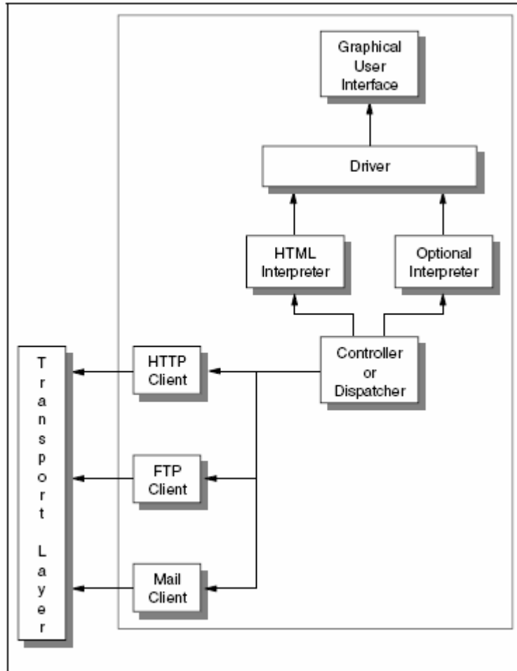
Gambar 13.4 Struktur Web Browser
