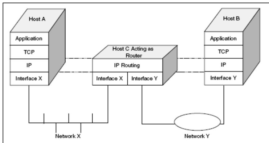
Gambar 6.1 Operasi routing sebuah pada IP
