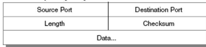
Gambar 7.2 Format Datagram UDP
