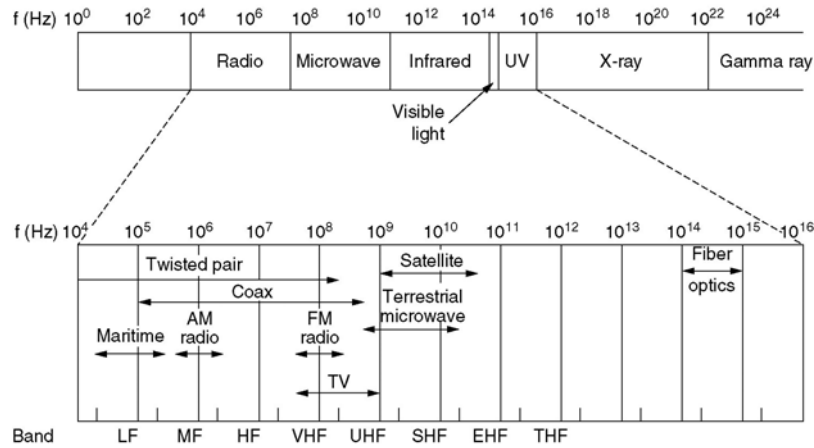
Gambar 3.30 Spektrum Elektromagnetik
