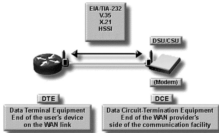
Gambar 3.17 Bentuk sambungan fisik perangkat WAN
