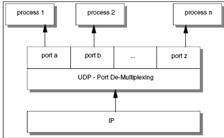
Gambar 7.1 Proses Demultiplexing berbasis port pada UDP
