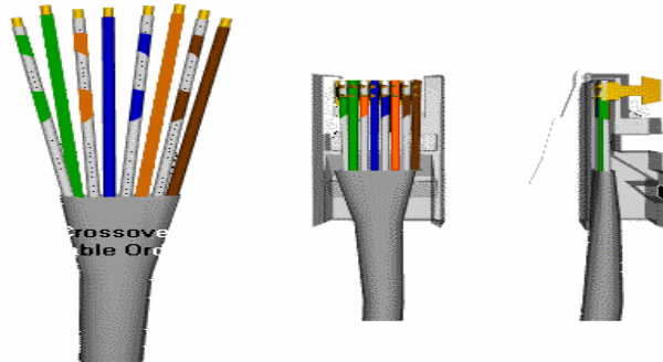
Gambar 3.28 TIA/EIA-586-A
