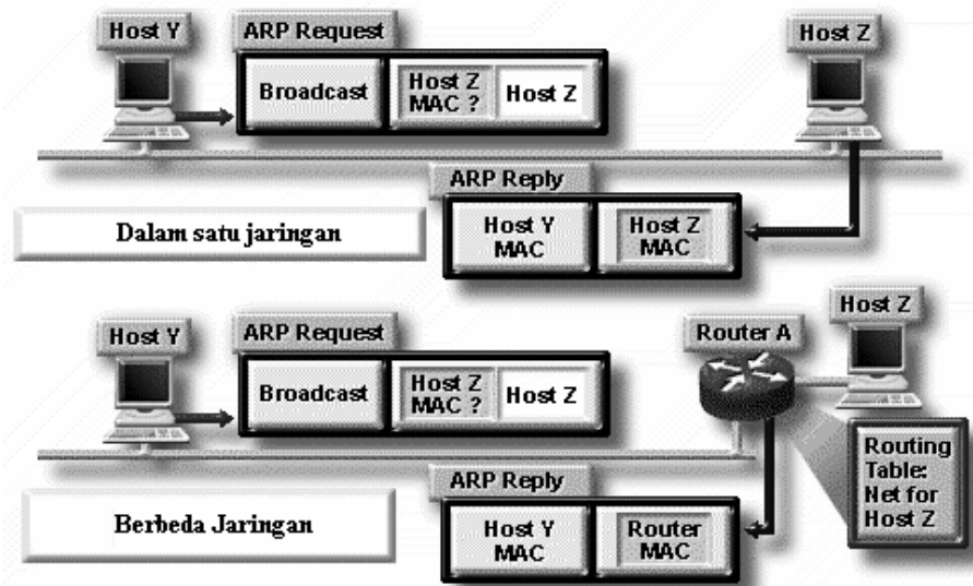
Gambar 5.2 Cara kerja protokol ARP
