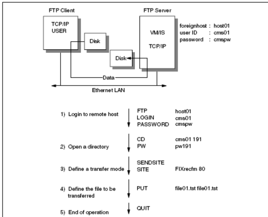
Gambar 11.2 FTP – Skenario FTP
