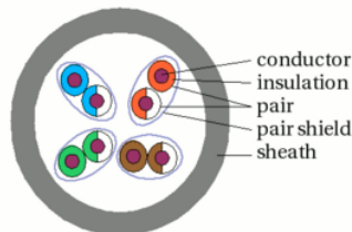
Gambar 3.24 STP
