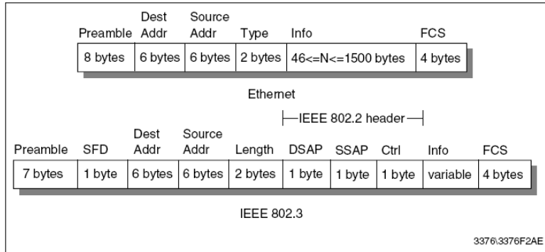
Gambar 3.5 Format frame untuk Ethernet dan IEEE 802.3
