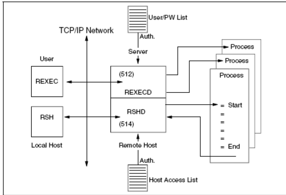
Gambar 10.2 Prinsip REXEC dan REXECD
