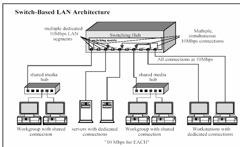
Gambar 3.12 Cara kerja Switch
