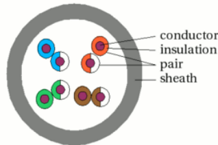
Gambar 3.23 UTP
