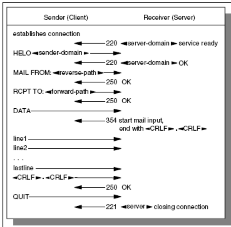
Gambar 12.3 Aliran SMTP
