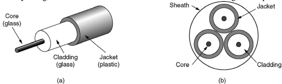
Gambar 3.29 (a) Tampak samping, (b) FO dengan 3 core
