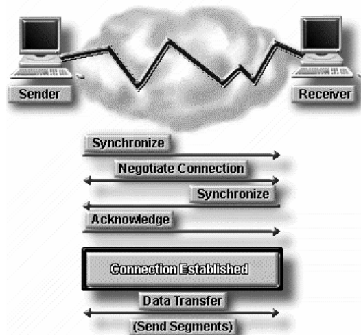
Gambar 2.6 Proses pembentukan koneksi
