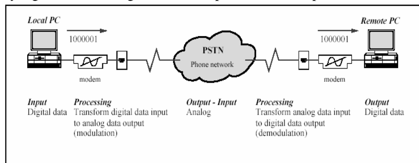
Gambar 3.19 Koneksi menggunakan Modem
