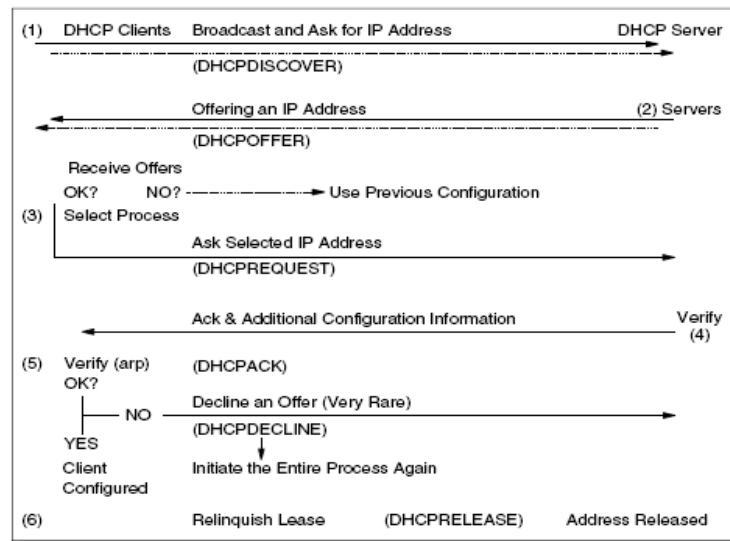
Gambar 5.3 Interaksi DHCP client dan DHCP server
