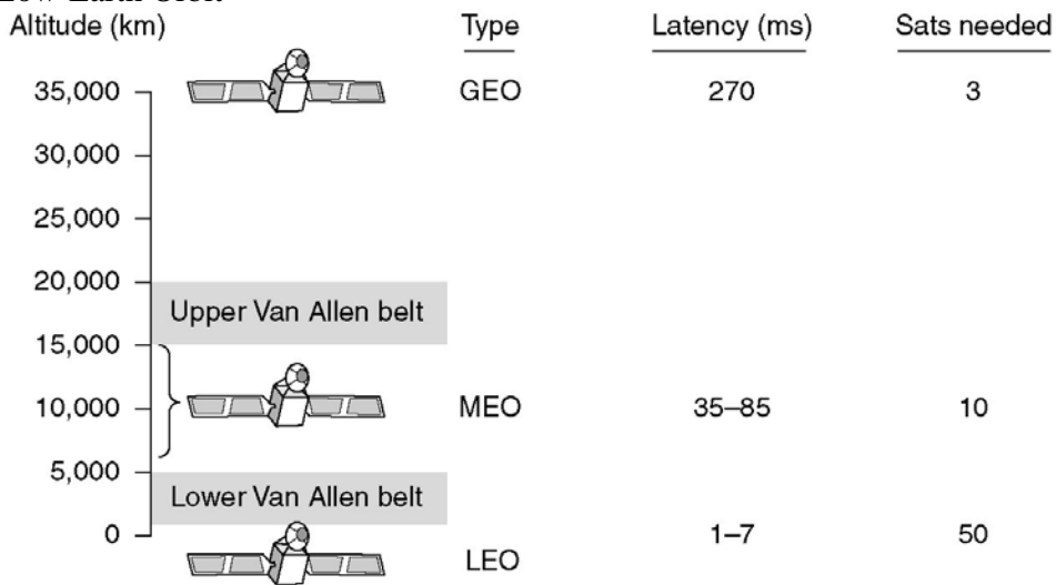
Gambar 3.34 Komunikasi Satelit
